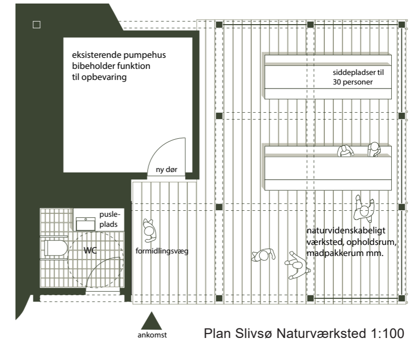
Plan Slivso Naturværksted 1:100
