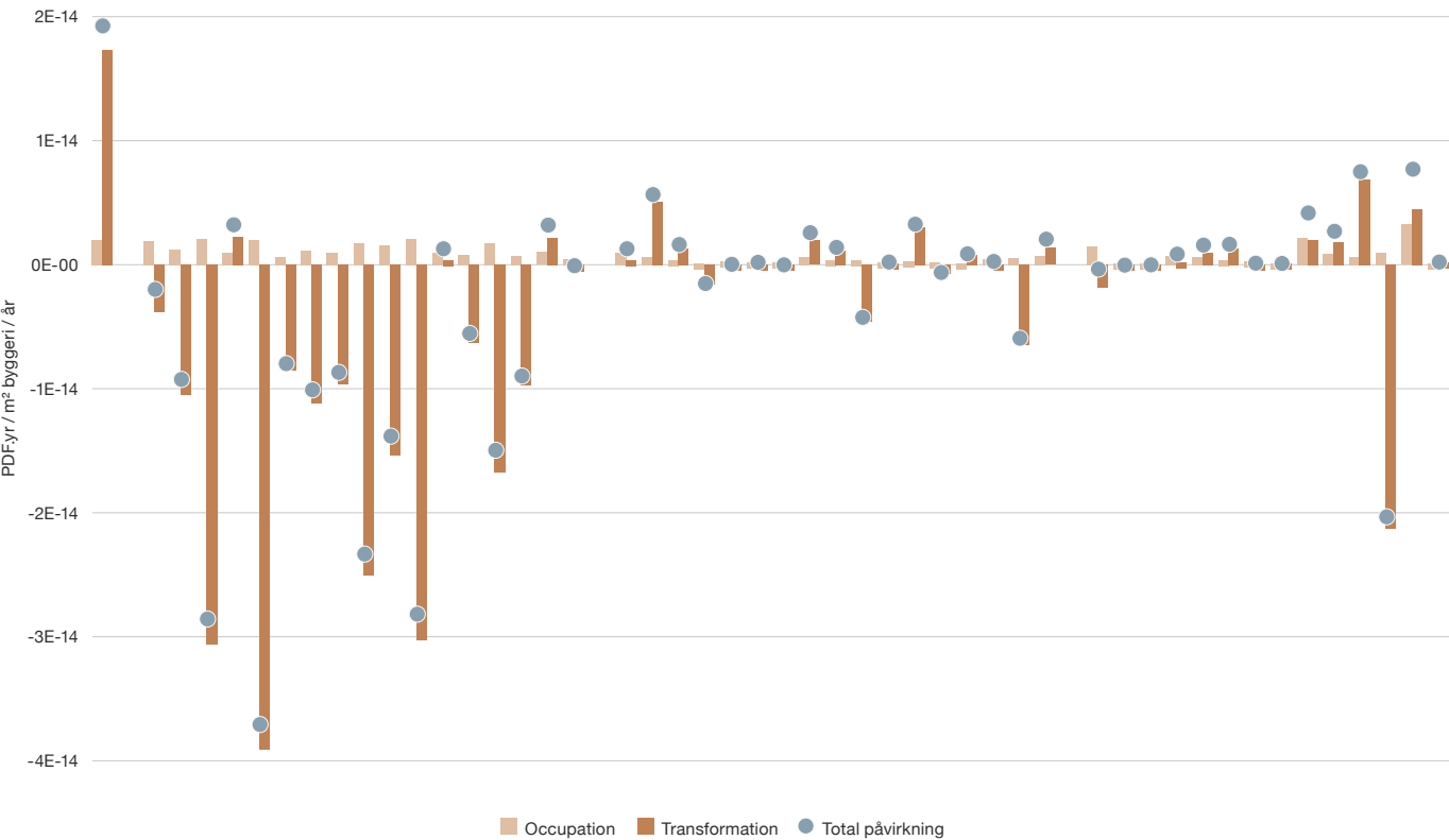
Figur 47: Casebibliotektets samlede biodiversitetspåvirkning på byggefeltet, samt bidrag fra occupation og transformation
