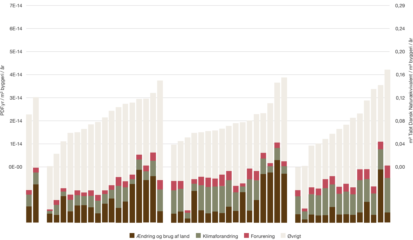
Figur 30: Casebibliotekets biodiversitetspåvirkning i værdikæderne, fremhævet for træ, beton og metal, fordelt på biodiversitetspåvirkningens primære drivere
