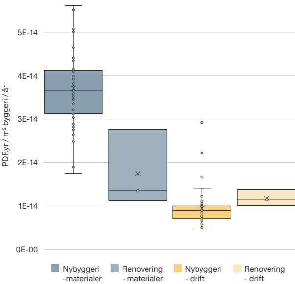
Figur 27: Casebibliotekets biodiversitetspåvirkning i værdikæderne, fordeling indenfor nybyggeri og renovering, fordelt på materialer og energiforbrug
