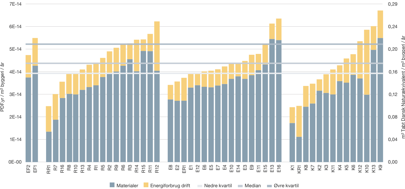
Figur 43: Casebibliotekets biodiversitetspåvirkning i værdikæderne, fordelt på materialer og energiforbrug, inklusiv forslag til bottom-up baseline værdier
