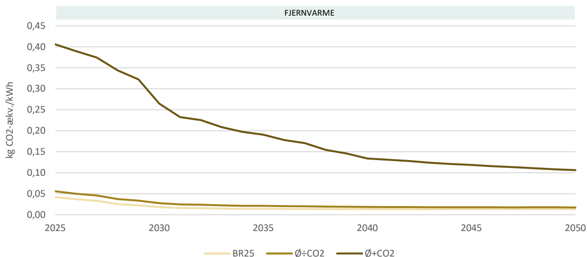
Figur 18 Sammenligning af scenarier for beregning af emissionsfaktor for fjernvarme - BR25, Ø±CO2 og Ø+CO2
