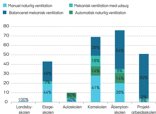
Figur 7: Fordeling af antallet af klasseværelset ift. ventilationsform opdelt efter bygningstypologi. I alt 250 klasseværelser.
