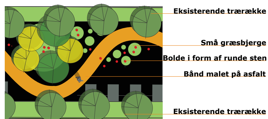
Plan 1:500 og snit 1:125
