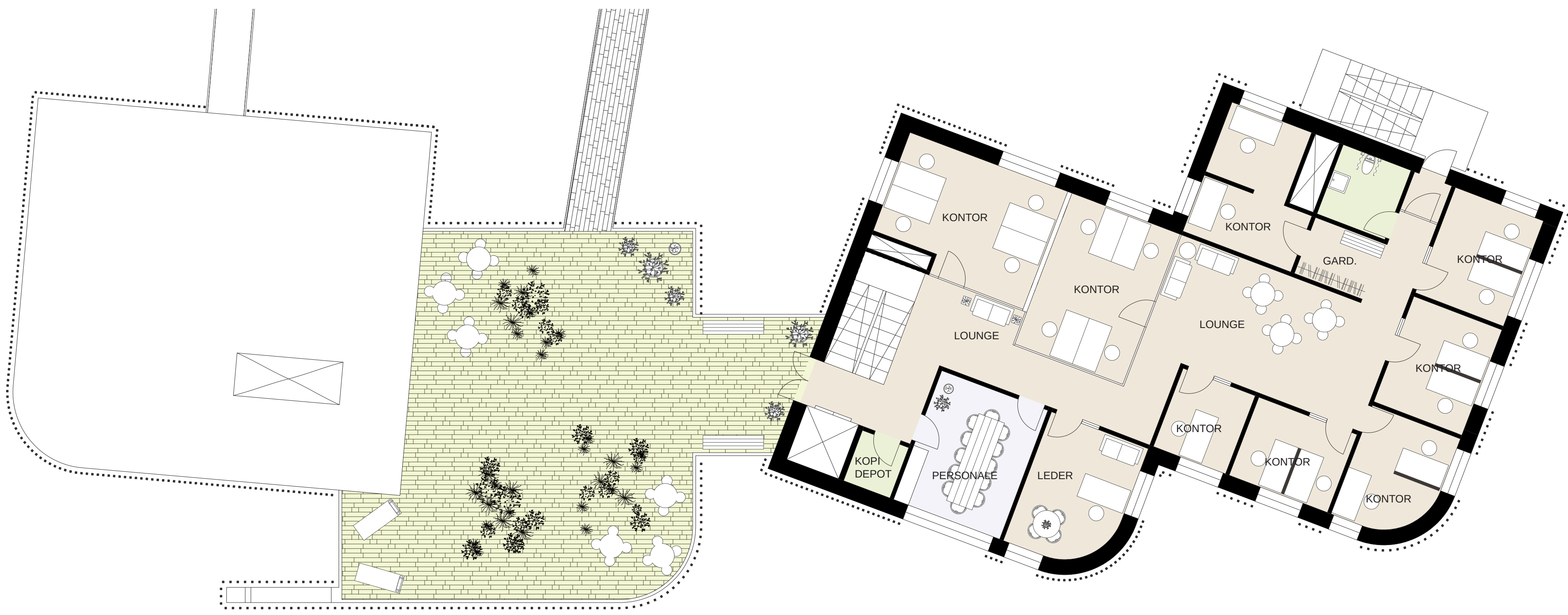
Plan niv. 03 1:100
