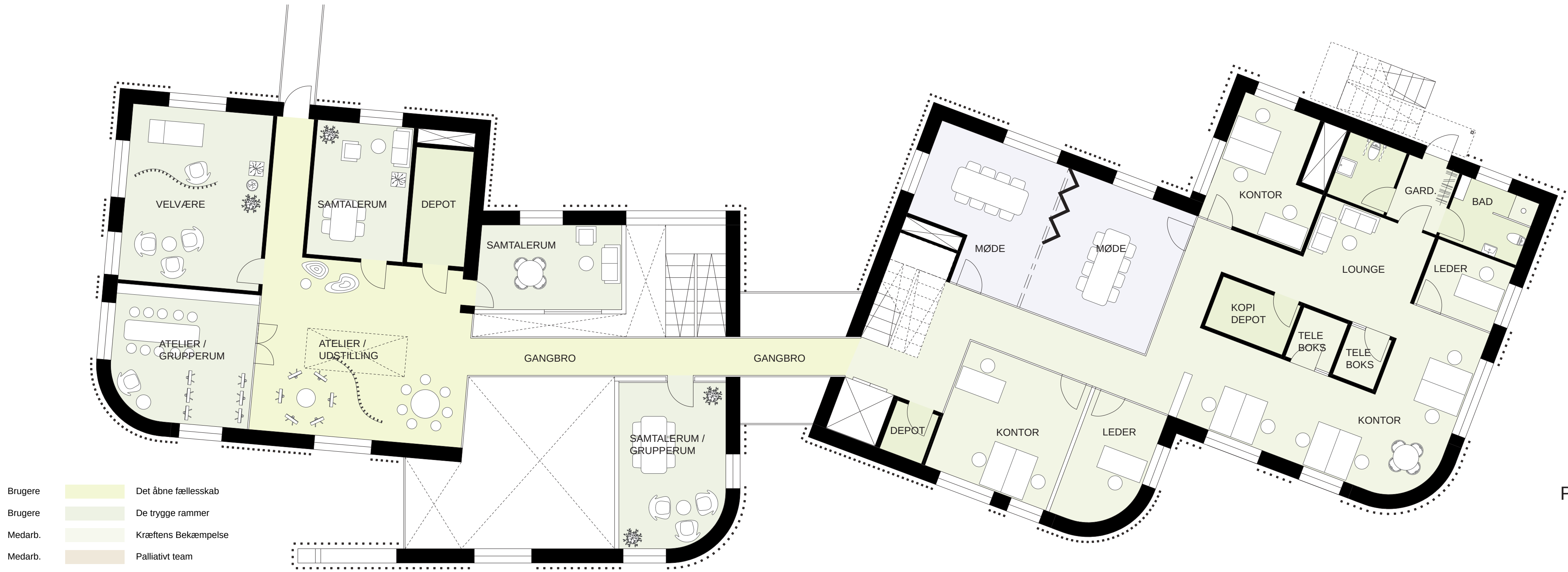
Plan niv. 02 1:100
