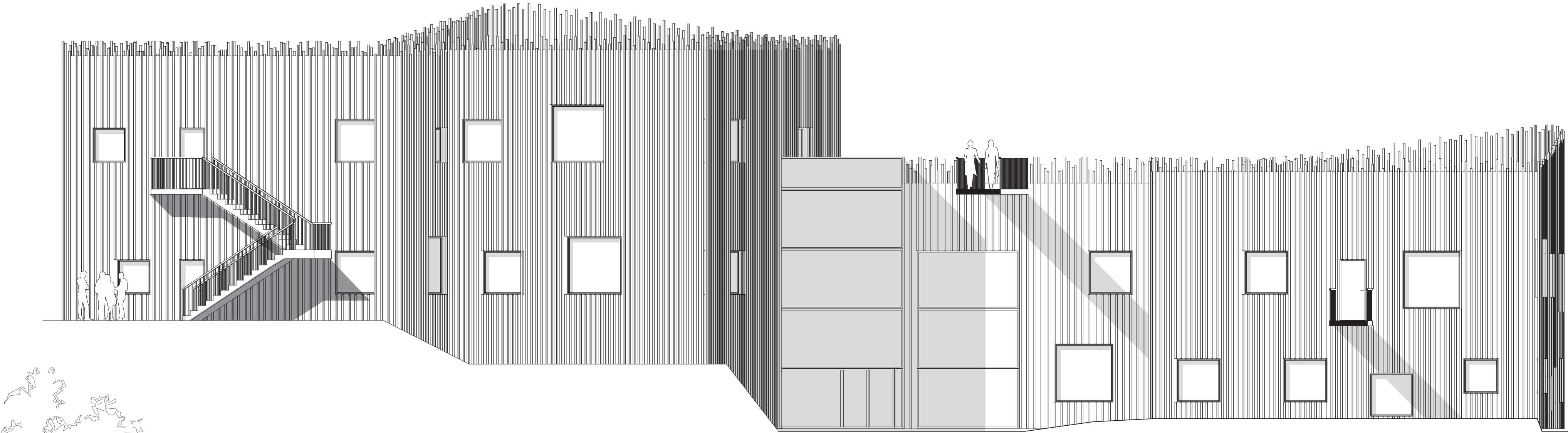
opstalt nord 1:100
