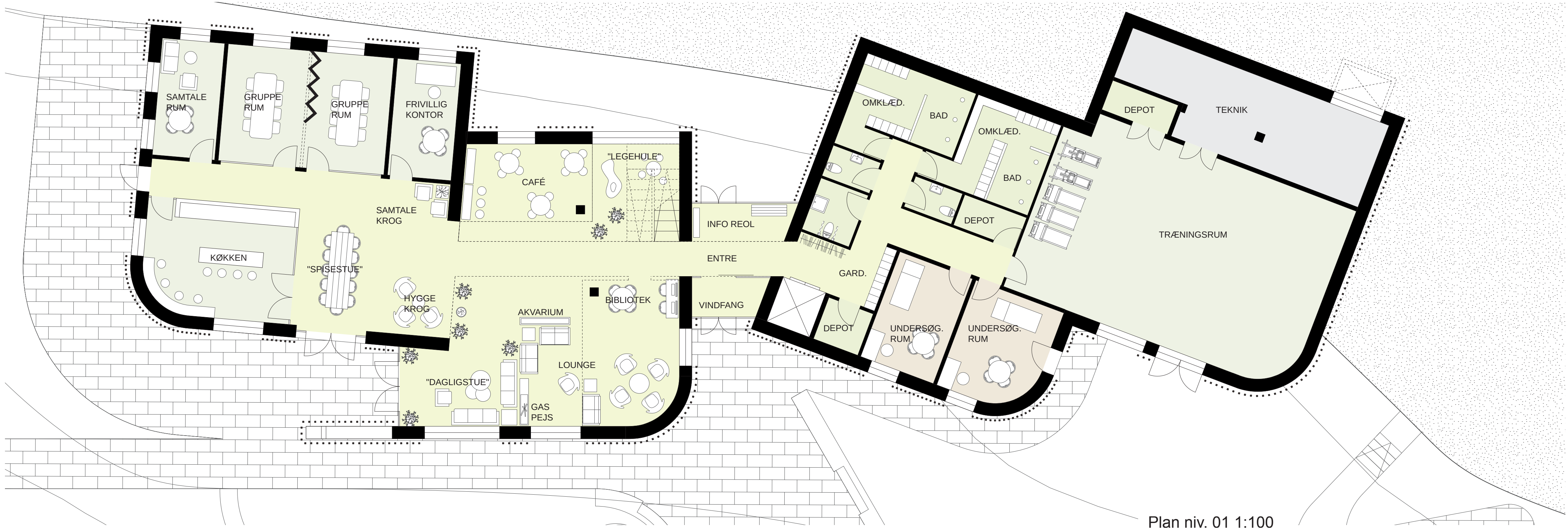
Plan niv. 01 1:100
