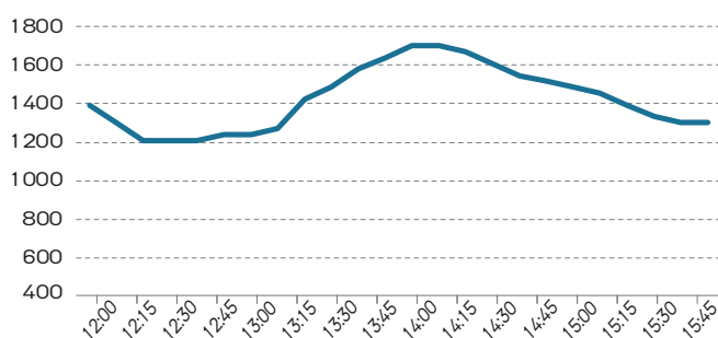
Figur 15: \text{CO}_2 -koncentration før initiativ.
