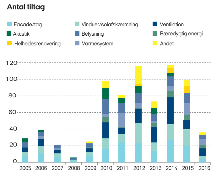
Figur 4: Renoveringstiltag fordelt på år [366 skoler, år 2016 er ikke repræsentativ].
